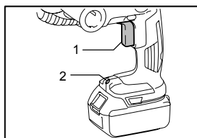
1. Gâchette 2. Lampe
